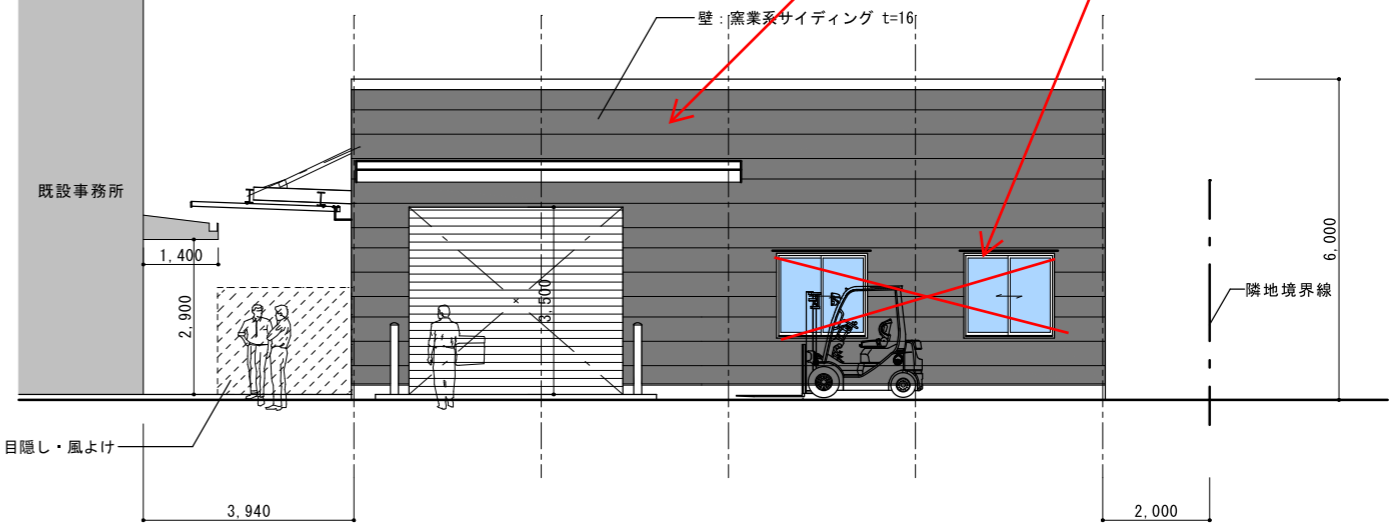
南側立面図 1/100
