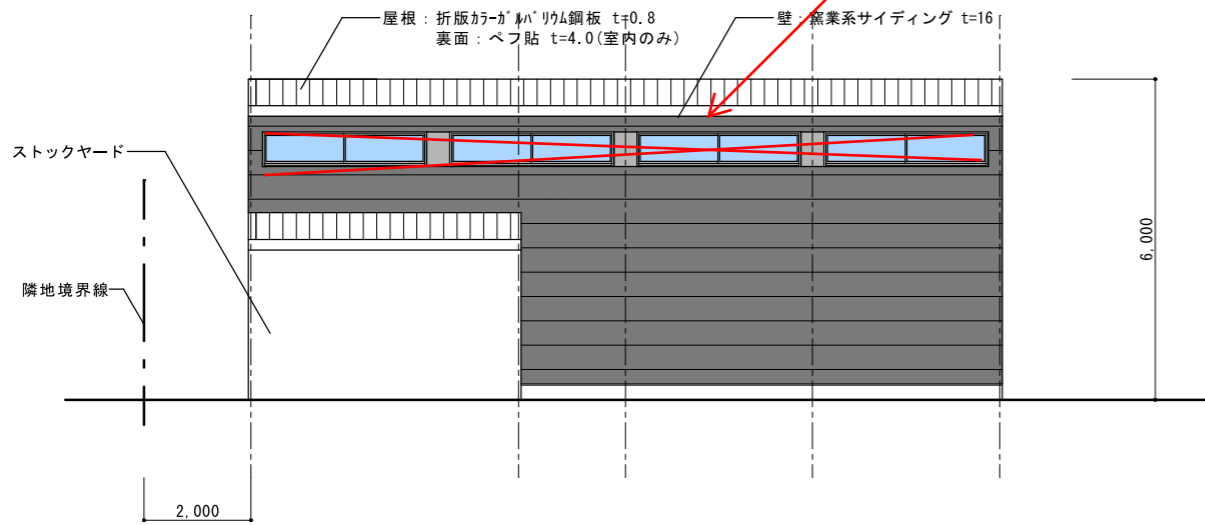
北側立面図 1/100
