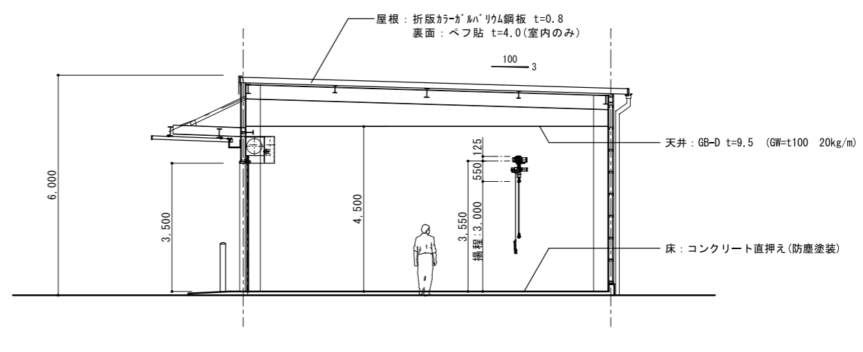
断面図 1/100
