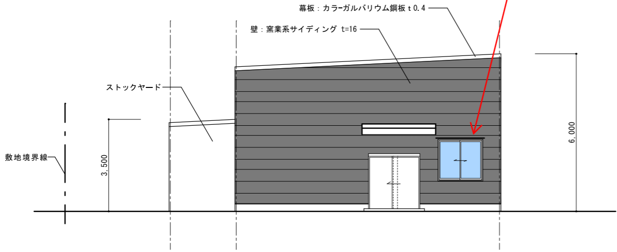
西側立面図 1/100
