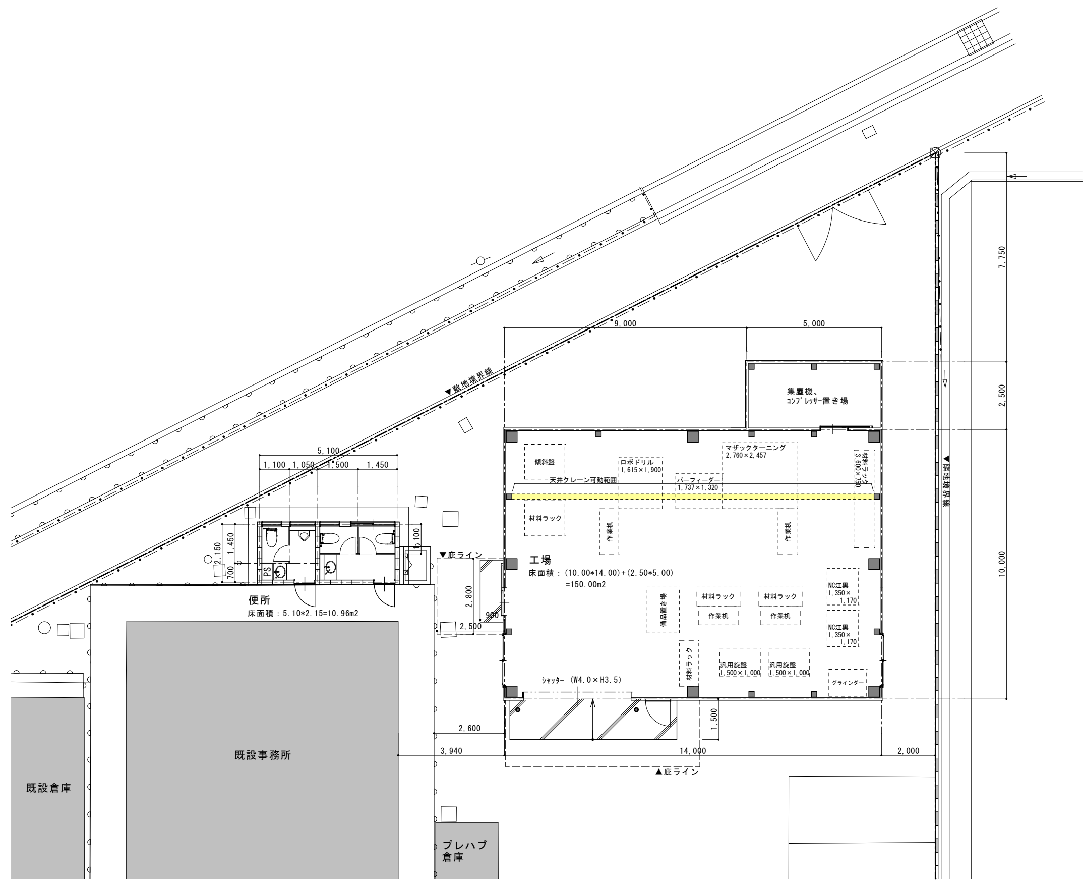
平面計画図 1/100
