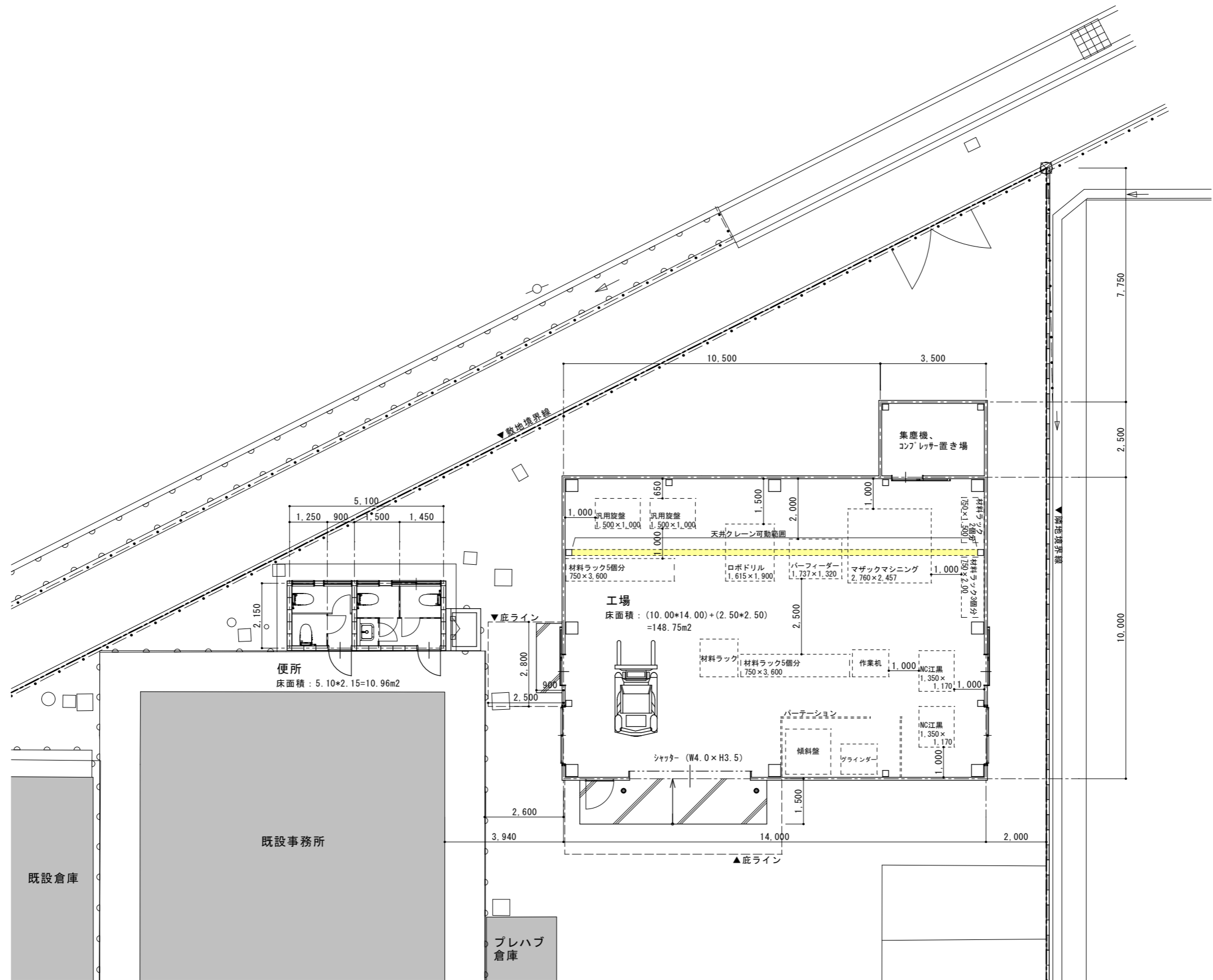
平面計画図 1/100
